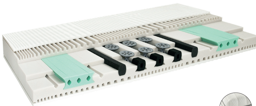
Softschaum in der Schulterkomfortzone
